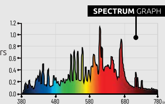
Spektrální graf 315W 3100K
