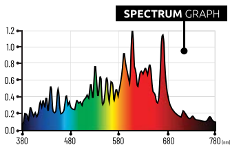
Spektrální graf 630W 3100K
